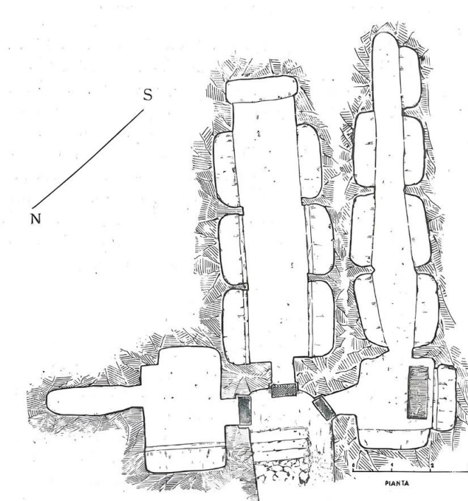
Pianta del sepolcreto: il vestibolo aperto verso nord-ovest e i tre ambienti ipogei (Morpurgo 1944-45, fig. 1).
